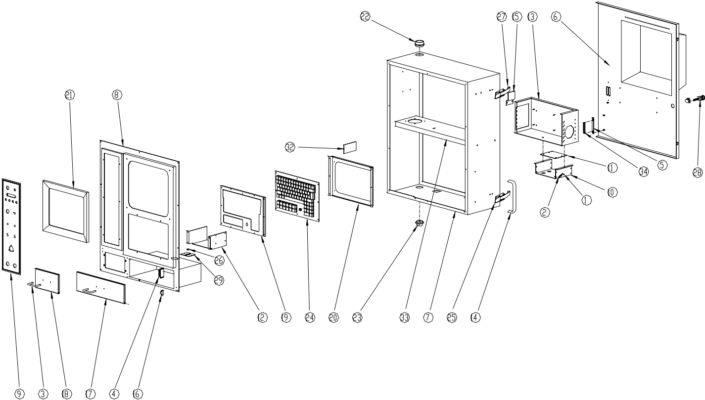
32MP PENDANT ASS
