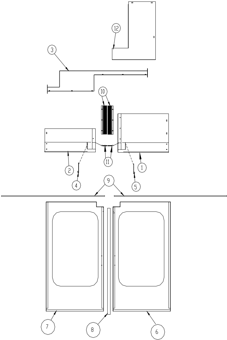
CHAIN HOIST SHEETMETAL 3020
