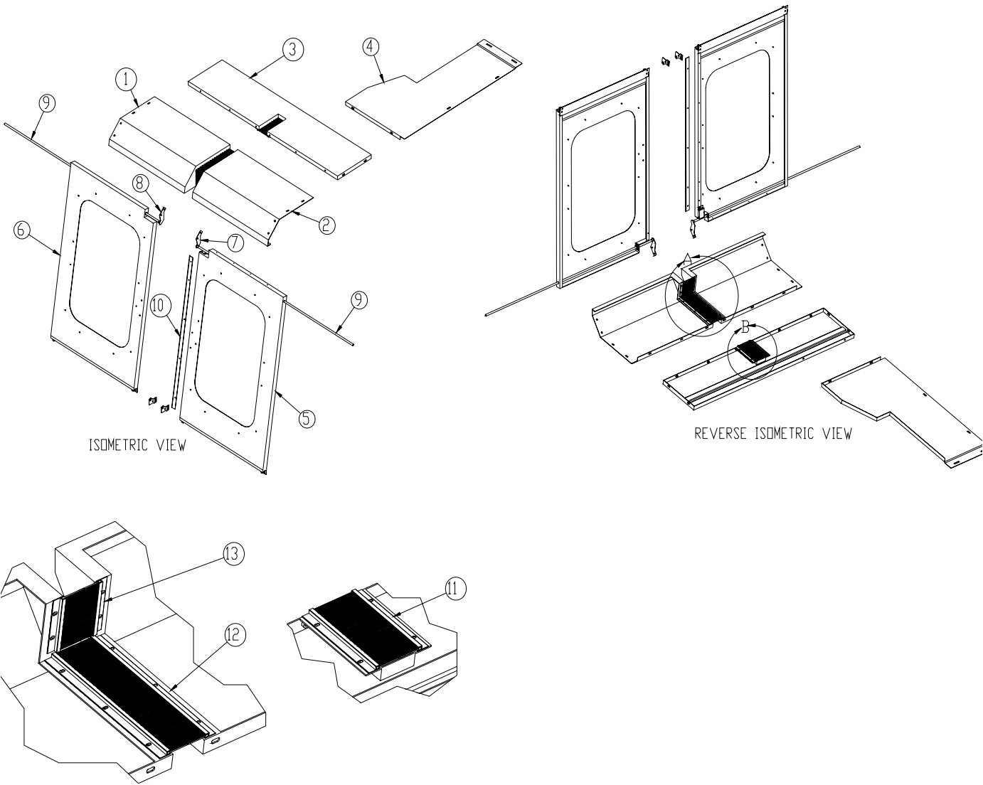
CHAIN HOIST SHEETMETAL 6535
